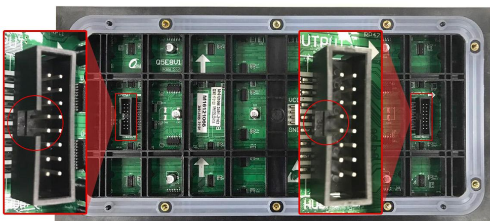
模组卡口
